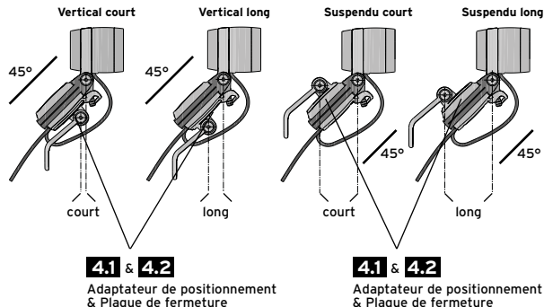
Fig. : quatre versions de montage du LEVAL Vertical - court | Vertical - long | Suspendu - court | Suspendu - long
