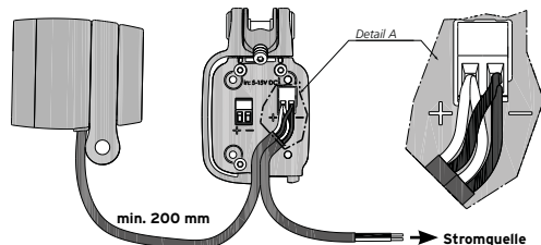
Abb.: Scheinwerfer und LEVAL zusammen an einer Stromquelle
