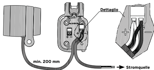
Figura: fanale e LEVAL allacciati assieme a una fonte di energia elettrica.
