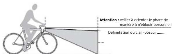
Fig. Exemple de réglage du phare
