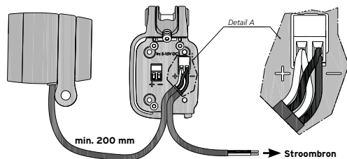
Afb.: Koplamp en LEVAL samen aan één stroombron
